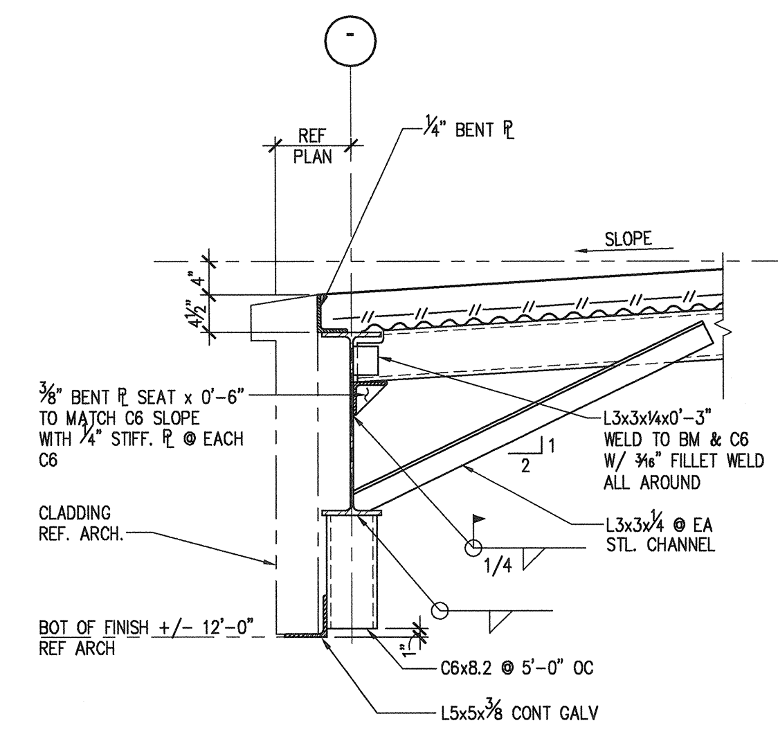
1 SCALE: 3/4\"/>
