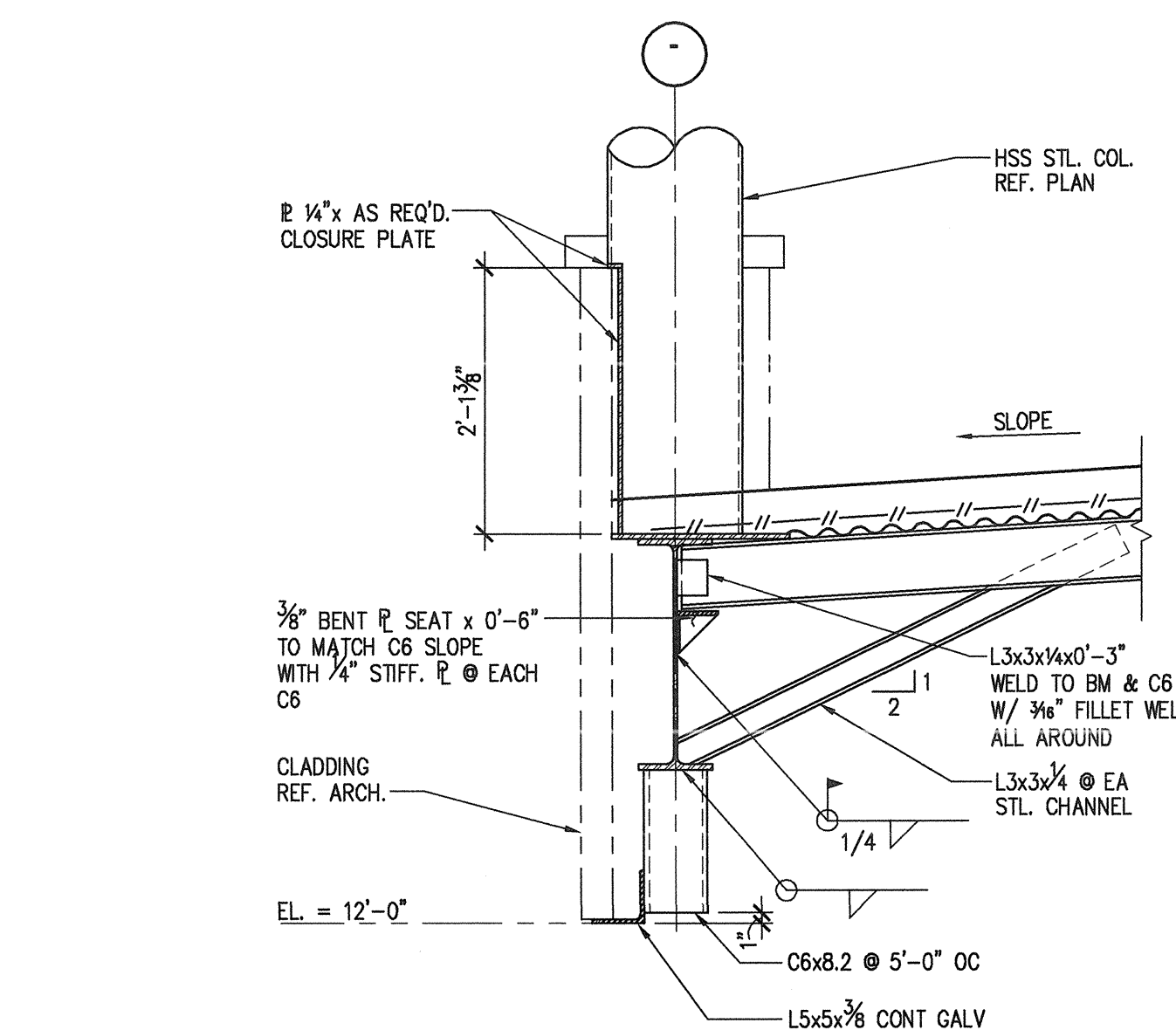
6 SCALE: 3/4\"/>
