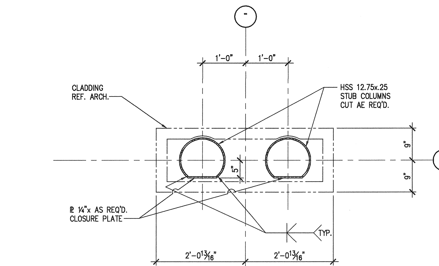
5 SCALE: 3/4\"/>
