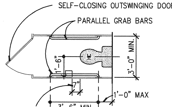
CRUTCH STALL Scale: 1/4"=1'-0"
