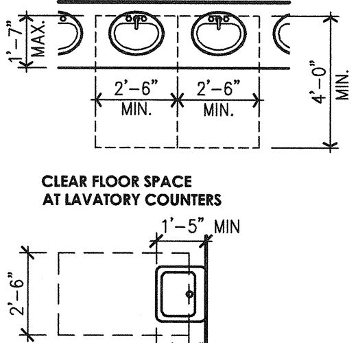
LAV. CLEARANCE Scale: 1/4"=1'-0"
